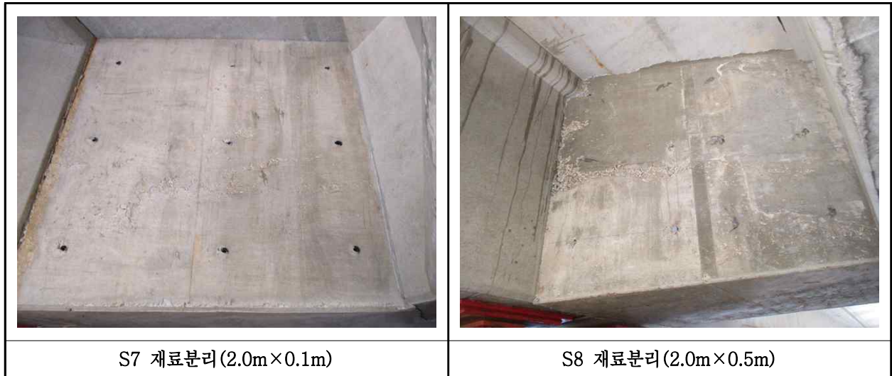
【사진 2.3.7】 가로보 손상현황
