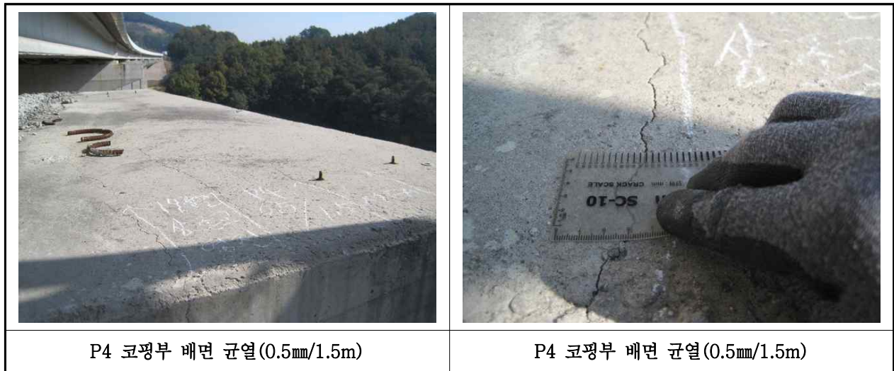
【사진 2.3.34】 교각 손상현황
