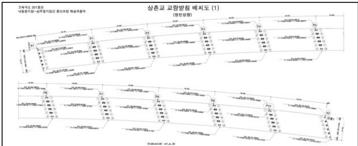
【그림 2.3.3】 교량받침 배치도
